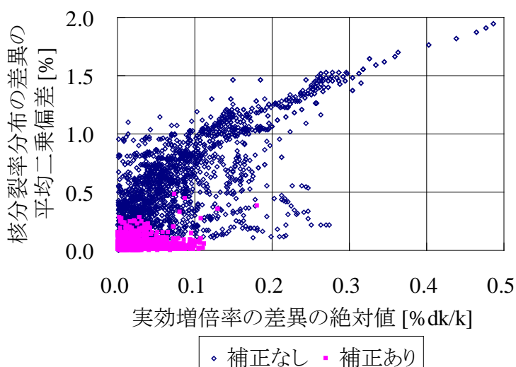
図 2 2 集合体体系における計算結果
