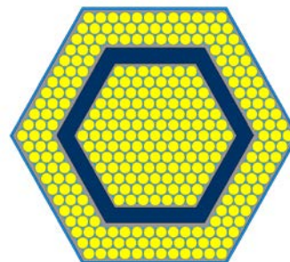
図 1 ZrH 付ブランケット集合体
