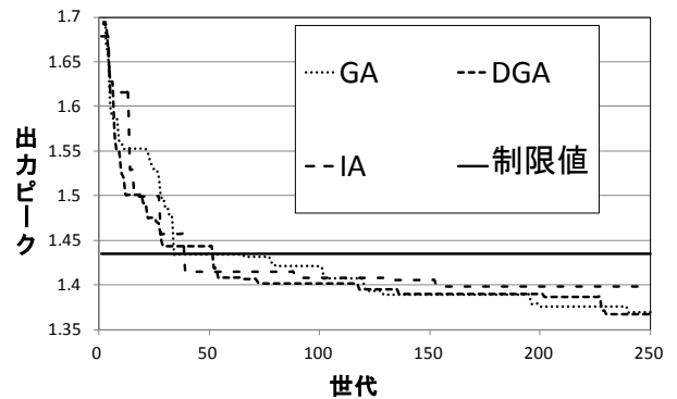
図 2 各最適化法のアルゴリズムの探索の様子
